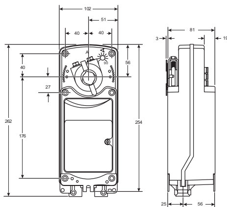
尺寸 (mm)
