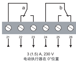
辅助开关(S)
