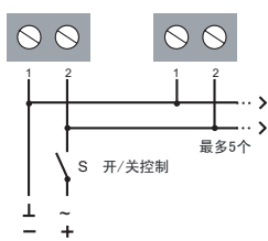
接线图
