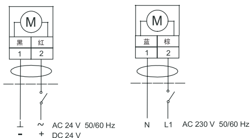
接线图
