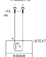
外部温度补偿
