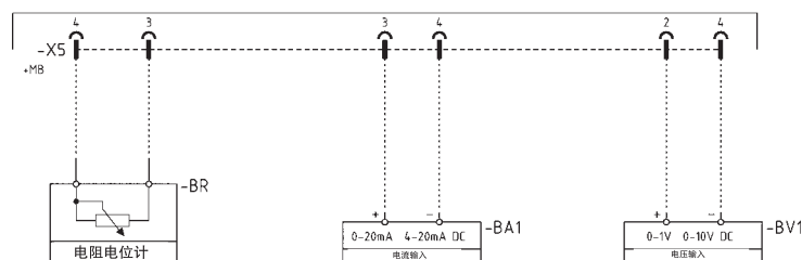
设定值输入及转换的信号类型
