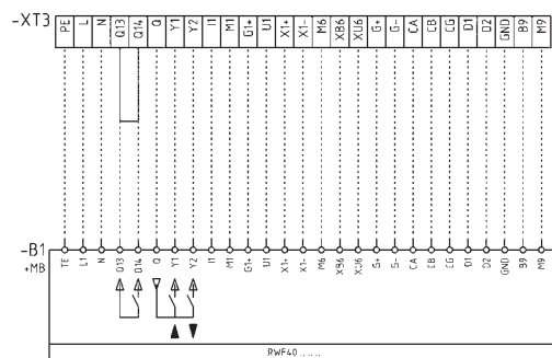
设定值输入及转换的信号类型
