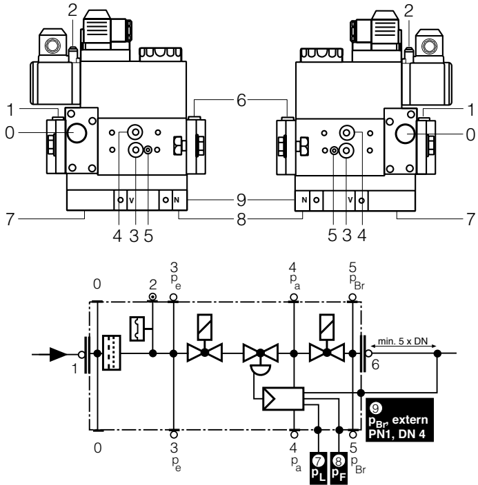
压力分接头，燃气流程图
