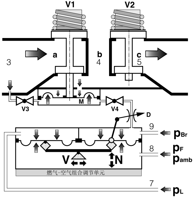
MB-VEF 原理图
