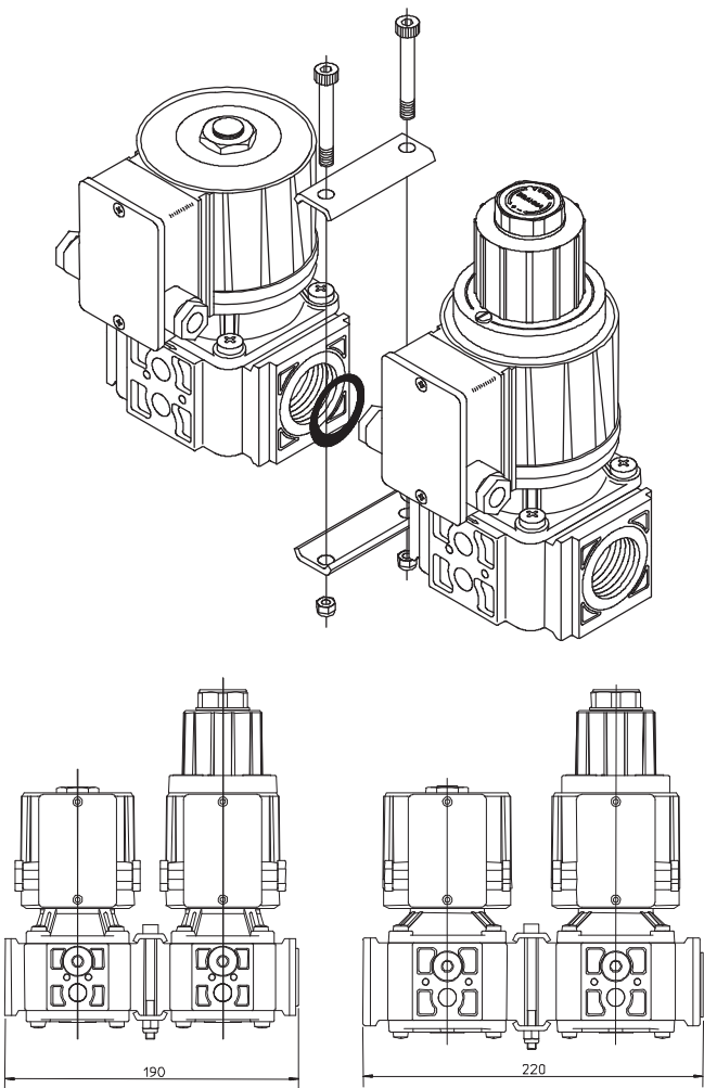
EG25*S-EG25*L阀组 EG30*S-EG30*L阀组
