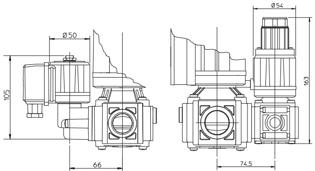
EG25旁通阀 Eg30旁通阀
