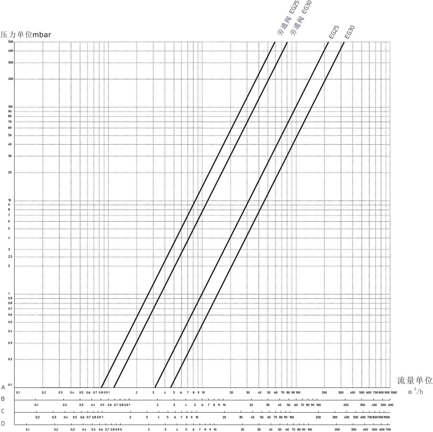
燃气阀流量曲线图
